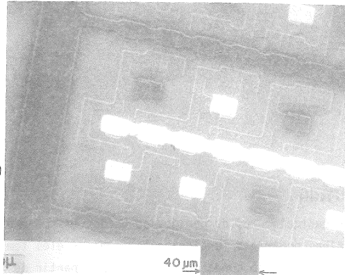
Fig. 12 - Fotografia do oscilador com alimentação mostrando o defeito (transistor defeituoso) (LAMM-UFRGS)
