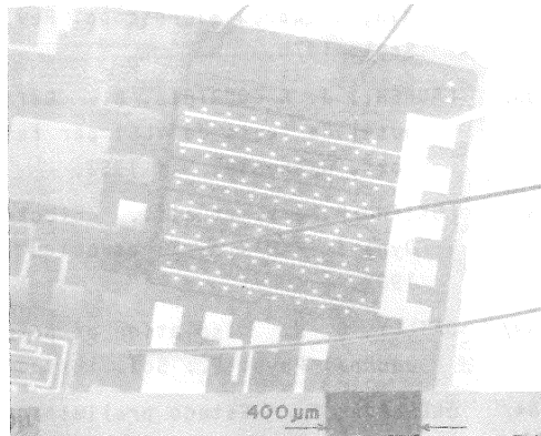
Fig. 10 - Fotografia do oscilador com alimentação mostrando o contraste por tensão nas linhas de alimentação (LAMM-UFRGS)
