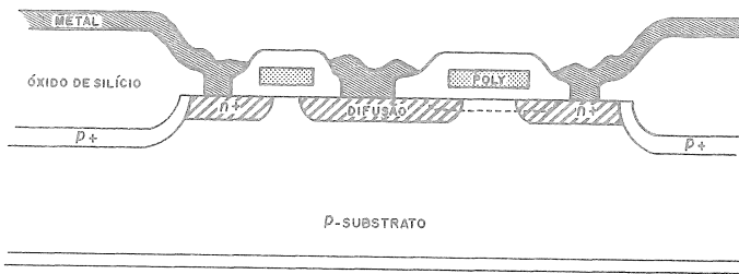
Fig. 2 - Vista de perfil de um inversor NMOS
