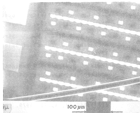
Fig. 11 - Fotografia do oscilador com alimentação mostrando a sequência de partes claras e escuras interrompida. (LAMM-UFRGS)
